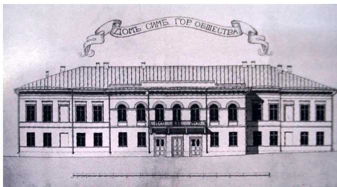
Фасад Дома Симбирского городского общества. Чертеж И. О. Бека.
